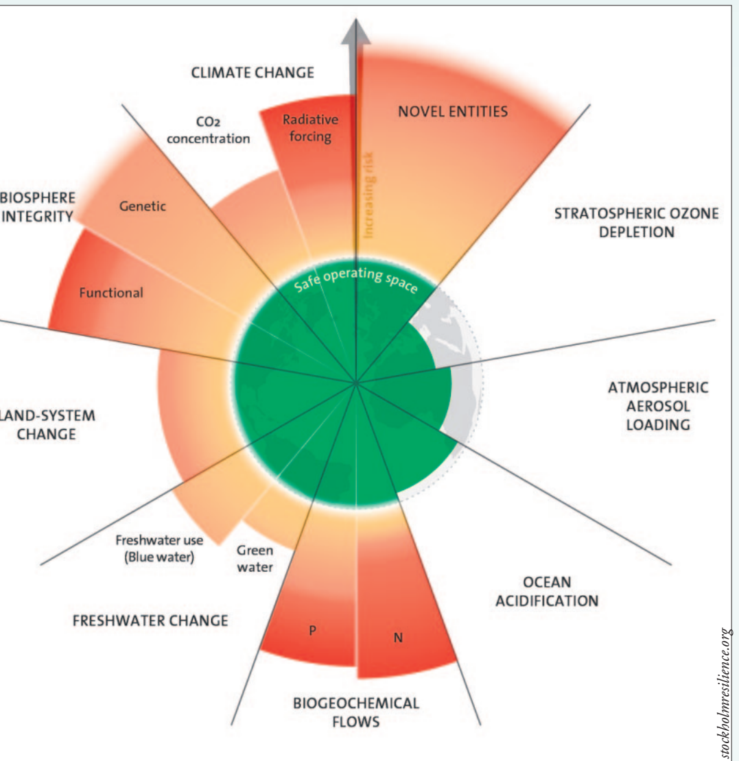
Schéma indiquant les limites planétaires et leur niveau de dépassement:
